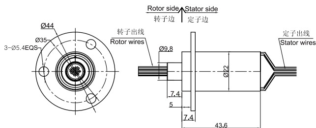
MC400图纸
