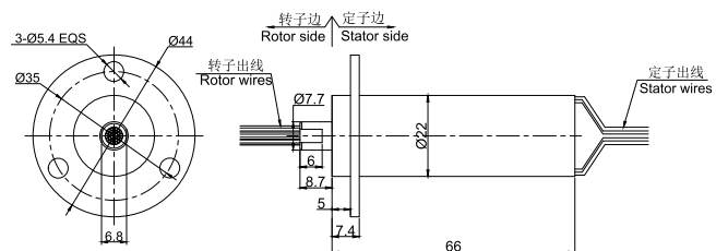
MC573-IP65 图纸
