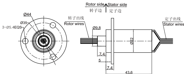
MC400图纸
