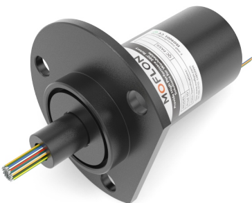
MC400-FL06图片
