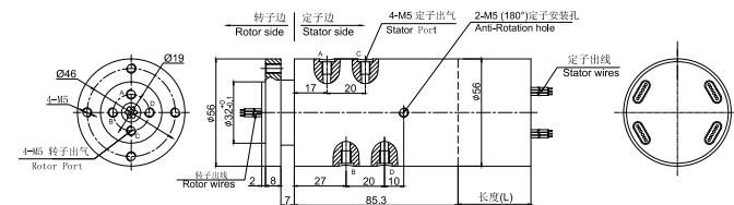
MAPH400-02 尺寸图
