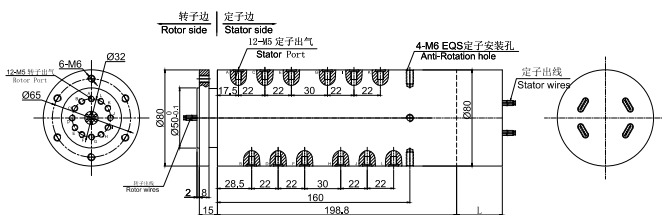
▼ MAPH1200-01气电一体 尺寸图
