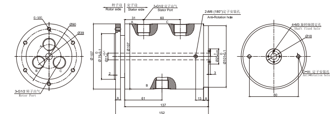
▼ MAPH300-05气电一体 尺寸图
