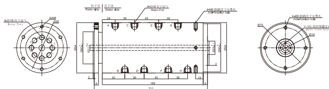
▼ MAPH800-02气电一体 尺寸图
