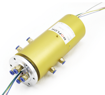
4进4出，G1/8接头
