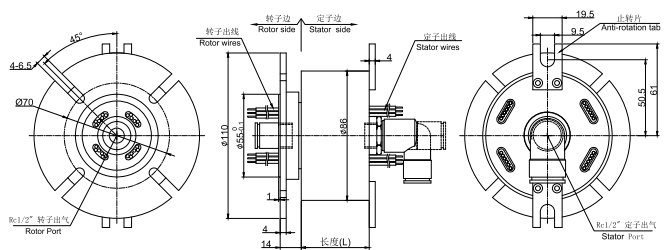
MAPH100-05 尺寸图
