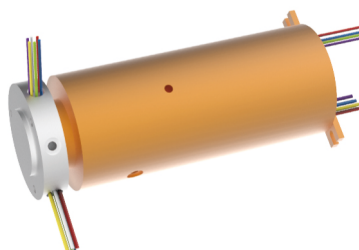
3进3出, G3/8接头
