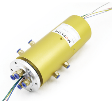
4进4出，M5接头
