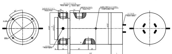
▼ MAPH200F-05气电一体 尺寸图
