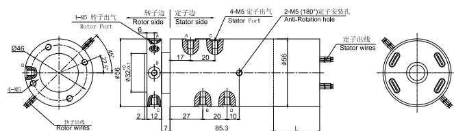
MAPH400F-02 尺寸图
