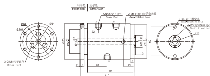
▼ MAPH300-02气电一体 尺寸图
