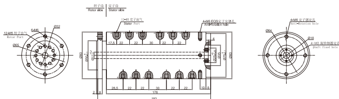
▼ MAPH1200-01气电一体 尺寸图
