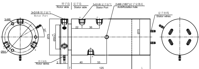
▼ MAPH300F-02气电一体 尺寸图
