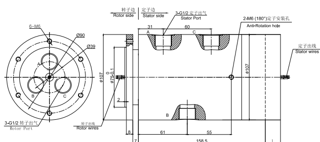
MAPH300S-05 尺寸图
