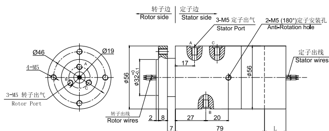
MAPH300S-02 尺寸图
