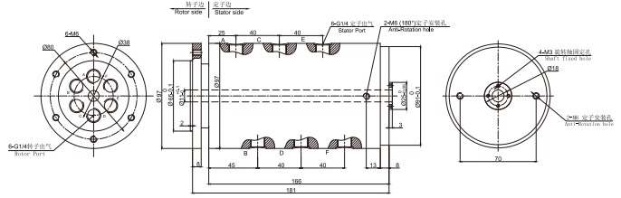
▼ MAPH600-03气电一体 尺寸图
