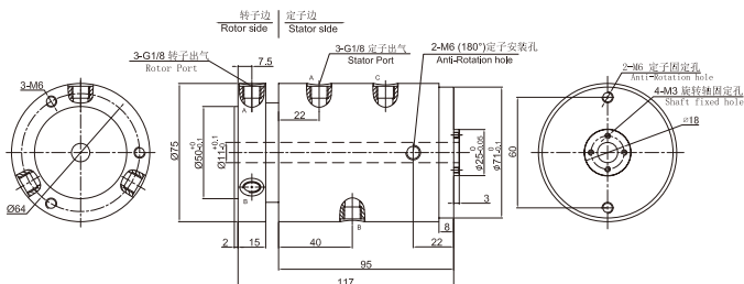
▼ MAPH300F-02气电一体 尺寸图
