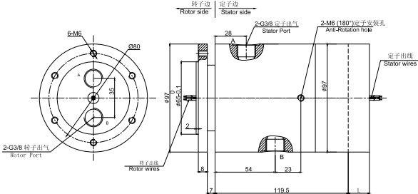
MAPH200S-05 尺寸图
