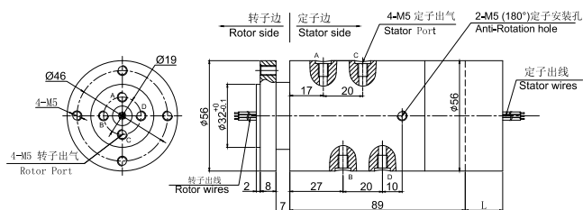
MAPH400S-02 尺寸图
