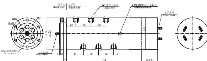
▼ MAPH600-02气电一体 尺寸图
