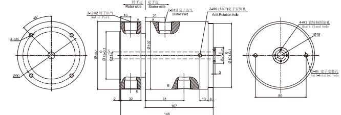
▼ MAPH200F-05气电一体 尺寸图
