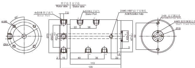
▼ MAPH400F-02气电一体 尺寸图
