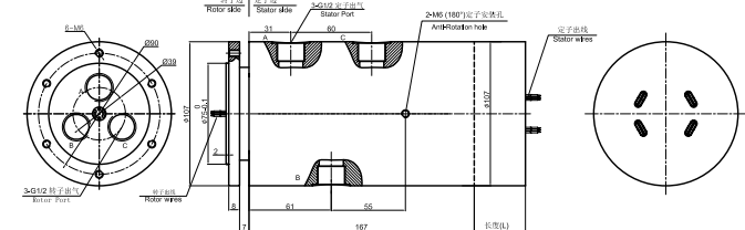
▼ MAPH300-05气电一体 尺寸图
