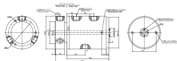
▼ MAPH300F-04气电一体 尺寸图
