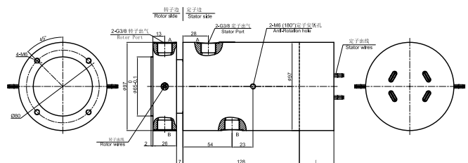
▼ MAPH200F-04气电一体 尺寸图
