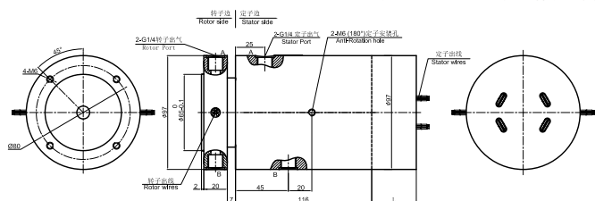
▼ MAPH200F-03气电一体 尺寸图
