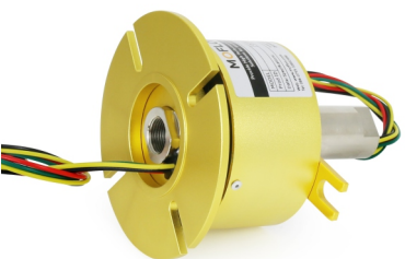
1进1出，G3/8接头
