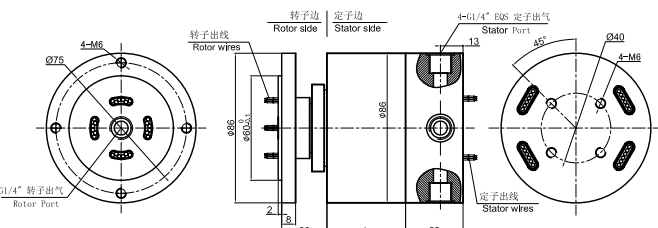
MAPH104-03 尺寸图
