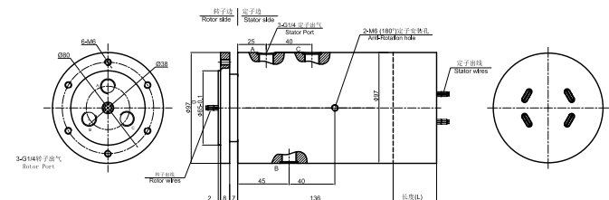
▼ MAPH300-03气电一体 尺寸图
