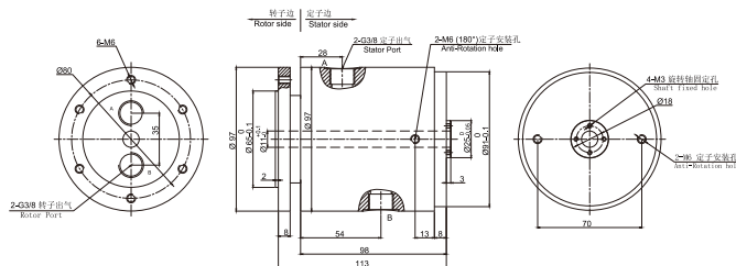
▼ MAPH200-04气电一体 尺寸图
