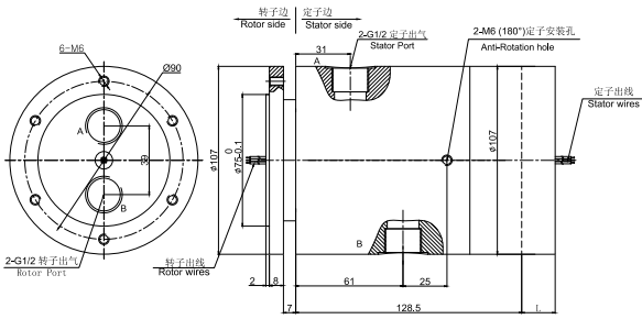
MAPH200S-05 尺寸图
