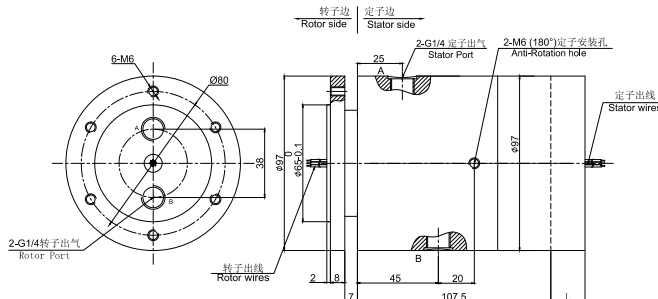
MAPH200S-03 尺寸图
