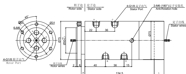
MAPH400S-03 尺寸图
