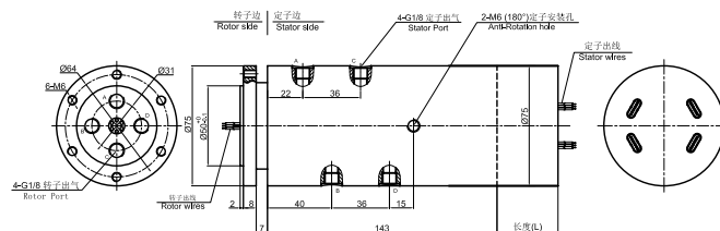
▼ MAPH400-02气电一体 尺寸图
