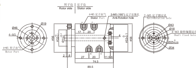
▼ MAPH400-01气电一体 尺寸图
