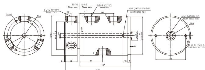
▼ MAPH300F-05气电一体 尺寸图
