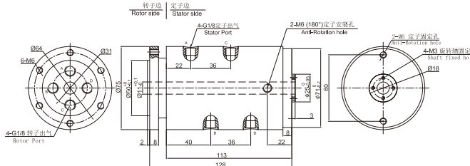
▼ MAPH400-02气电一体 尺寸图
