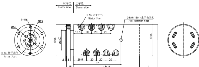
▼ MAPH800-01气电一体 尺寸图
