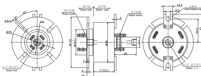
MAPH100-MK13W 尺寸图
