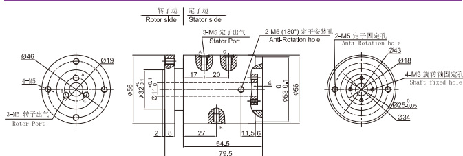
▼ MAPH300-01气电一体 尺寸图
