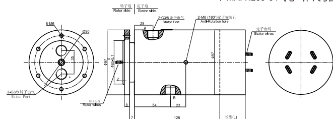
MAPH200-05 尺寸图
