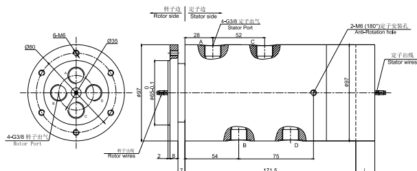
MAPH400S-05 尺寸图
