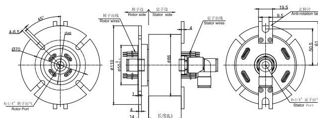
MAPH100-03 尺寸图
