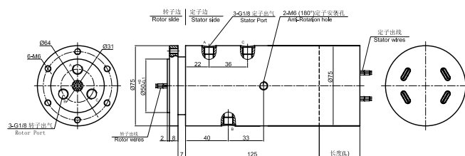
▼ MAPH300-02气电一体 尺寸图
