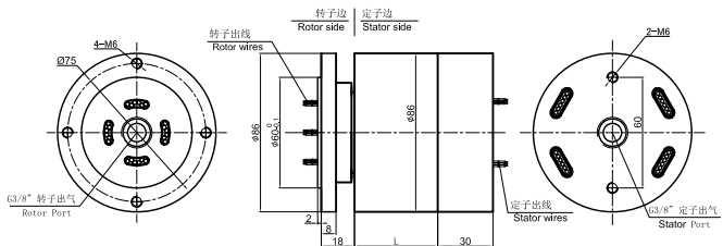
MAPH101-04 尺寸图
