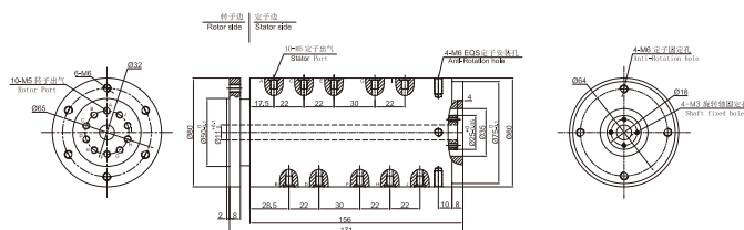
▼ MAPH1000-01气电一体 尺寸图
