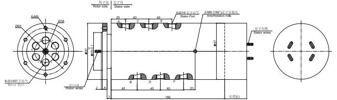
▼ MAPH600-03气电一体 尺寸图
