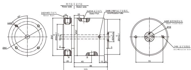
▼ MAPH200F-03气电一体 尺寸图
