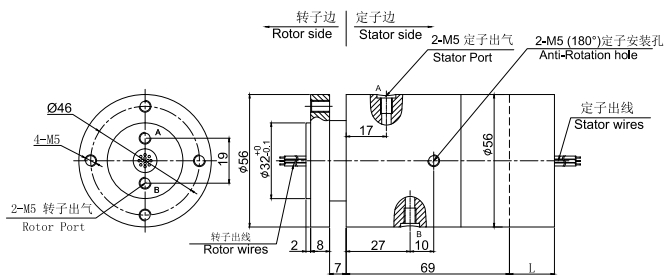
MAPH200S-02 尺寸图
