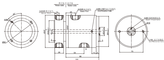
▼ MAPH200F-04气电一体 尺寸图
