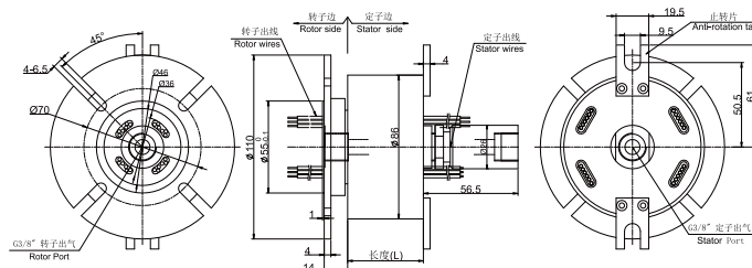
MAPH100-MK13W 尺寸图
