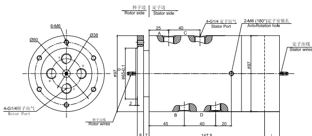
MAPH400S-03 尺寸图
