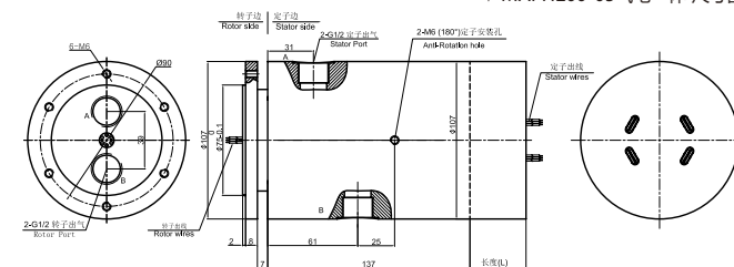
▼ MAPH200-05气电一体 尺寸图
