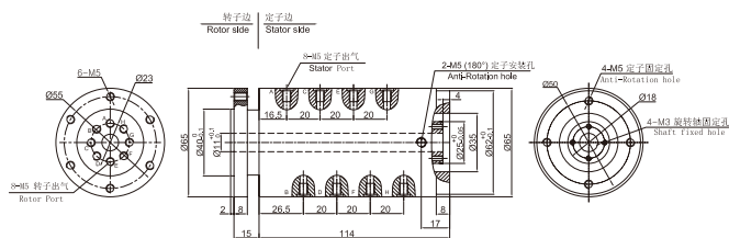
▼ MAPH800-01气电一体 尺寸图
