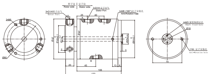
▼ MAPH300F-03气电一体 尺寸图
