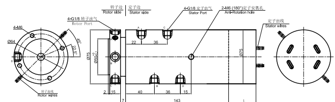
▼ MAPH400F-02气电一体 尺寸图
