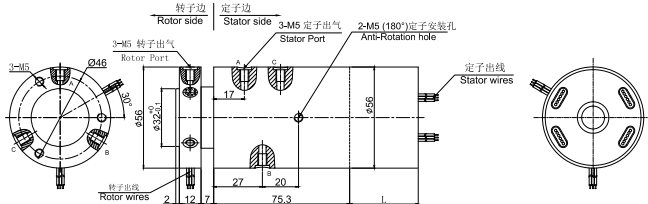
MAPH300F-02 尺寸图
