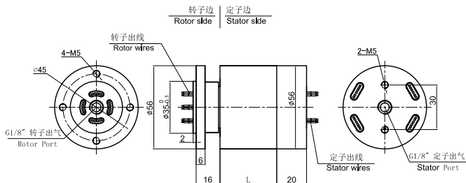
MAPH101-02 尺寸图
