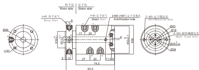
▼ MAPH400F-01气电一体 尺寸图
