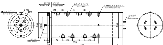
▼ MAPH800-02气电一体 尺寸图
