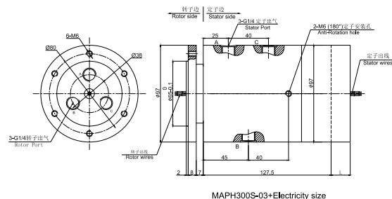
MAPH300S-03 尺寸图
