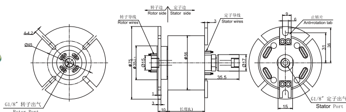
MAPH100-MK12W 尺寸图
